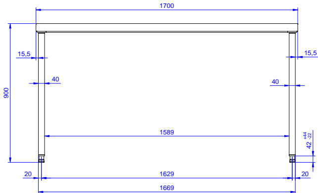
Front aanzicht
